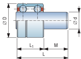
Type: 型号: 73-7-4
