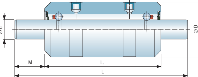
Type: 型号: 74-5-4
