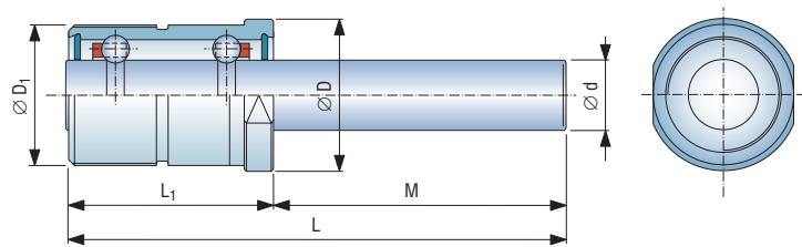
Type: 型号: 73-7-3
