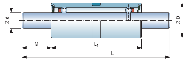
Type: 型号: 73-8
