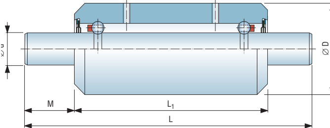
Type: 型号: 74-4-1
