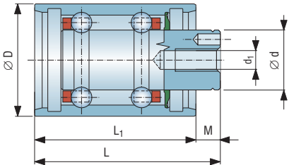
Type: 型号: 76-2-1
