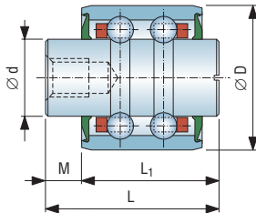
Type: 型号: 76-2-1
