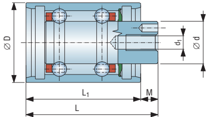
Type: 型号: 76-2-2
