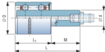
Type: 型号: 73-7-5
