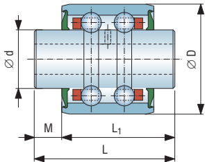
Type: 型号: 76-2-3
