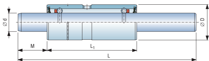
Type: 型号: 73-8
