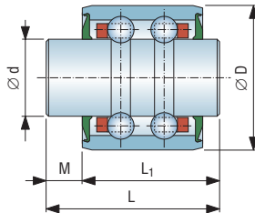
Type: 型号: 76-2-2
