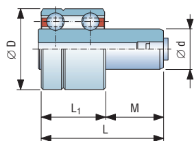
Type: 型号: 73-7-3
